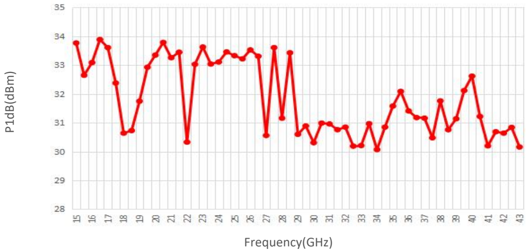
Pout@Pin
