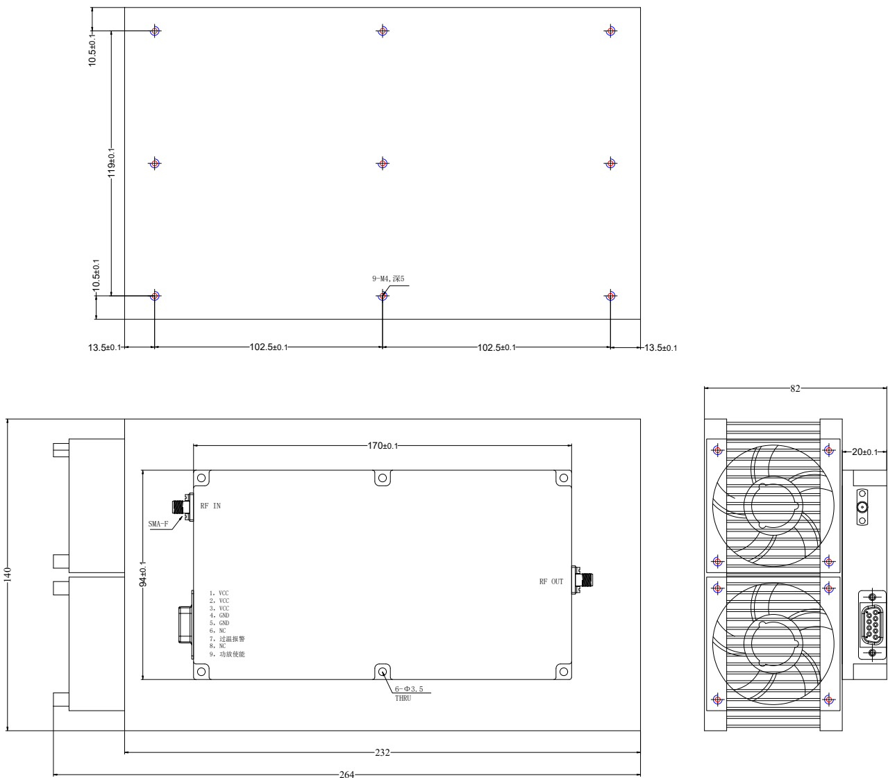
外形图 Outline Drawing: Unit:mm
