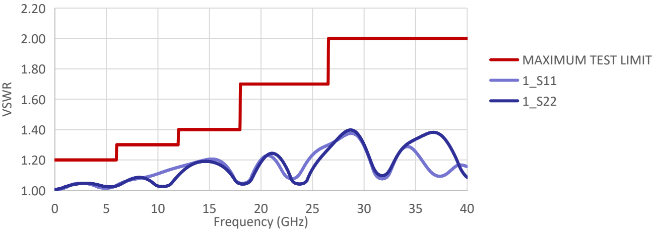
VSWR
