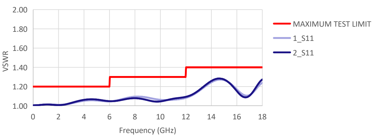
VSWR
