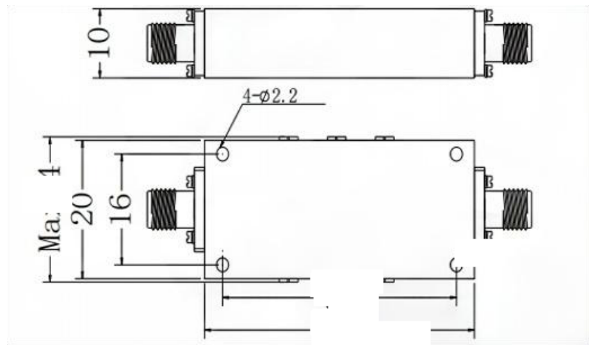
外形图 Outline Drawing: Unit:mm
