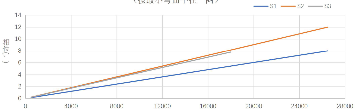
机械相位稳定性 (按最小弯曲半径一圈)
