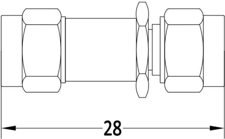
外形图 Outline Drawing: Unit:mm
