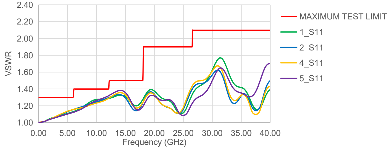
VSWR
